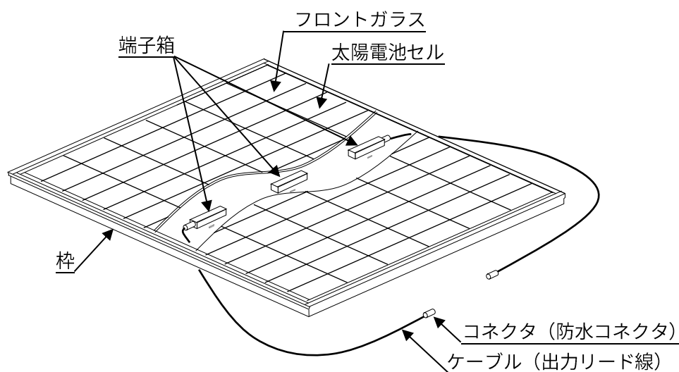
図 1. 太陽電池モジュール構成図
