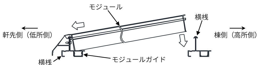
図 3-6. YSIII工法 モジュール固定図
