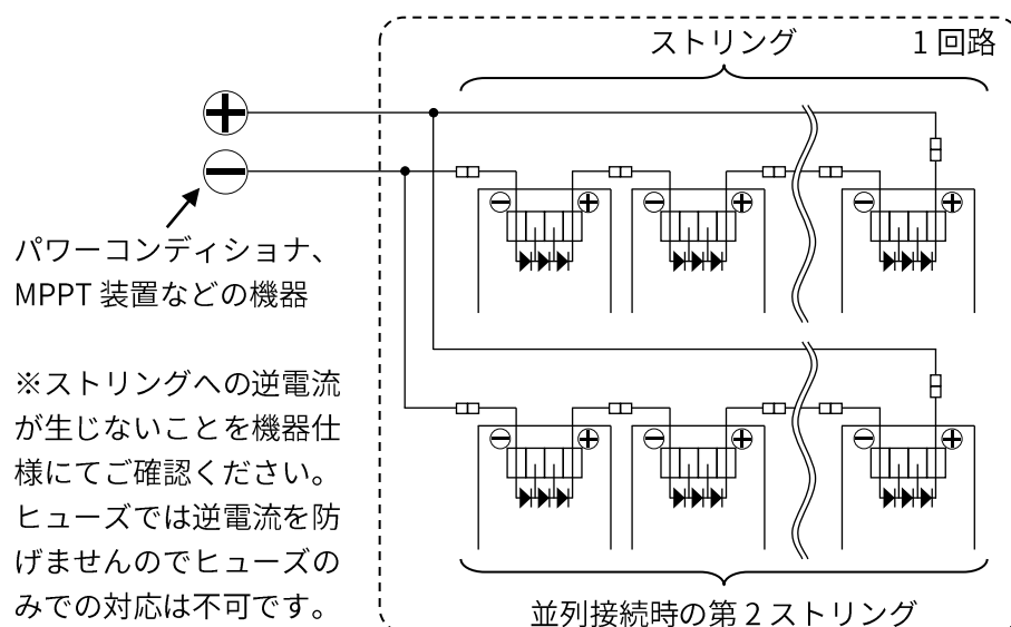
図 5. 2 本のストリングを並列接続する場合
