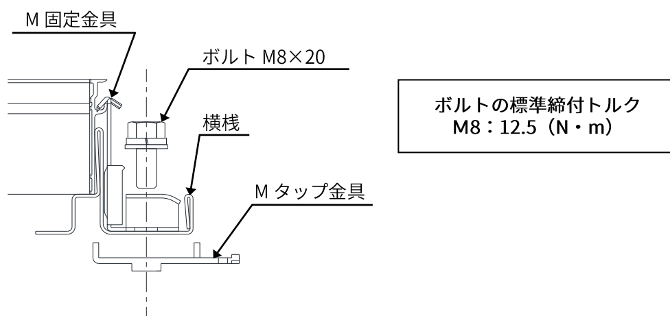
図 3-3. YS II 工法 金具の固定図
