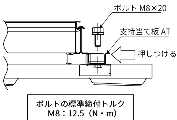
図 3-10. YSIII工法 横棧の固定図
