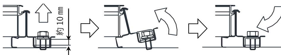
図 3-7. YSIII工法 モジュール固定手順
