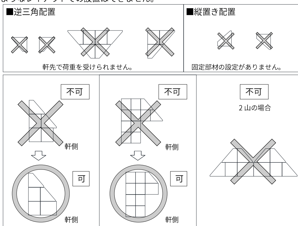
図5. 禁止レイアウト
