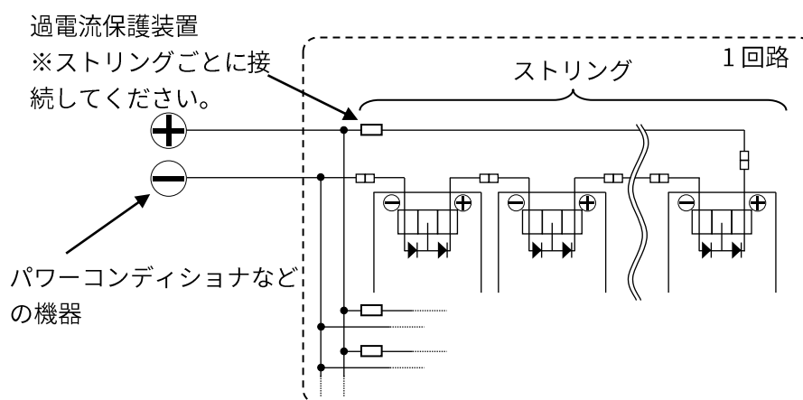
図 8. 3 本以上のストリングを並列接続する場合
