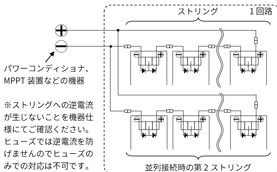
図 7. 2 本のストリングを並列接続する場合
