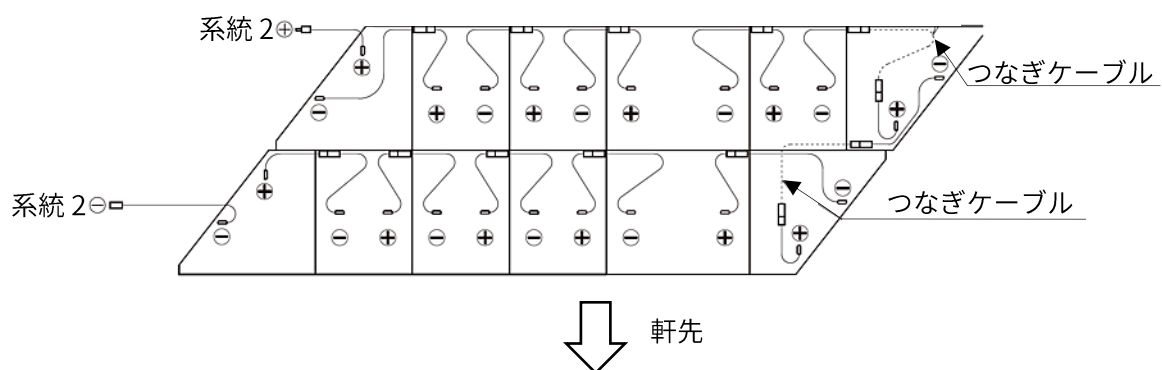
図4. つなぎケーブルの接続例
