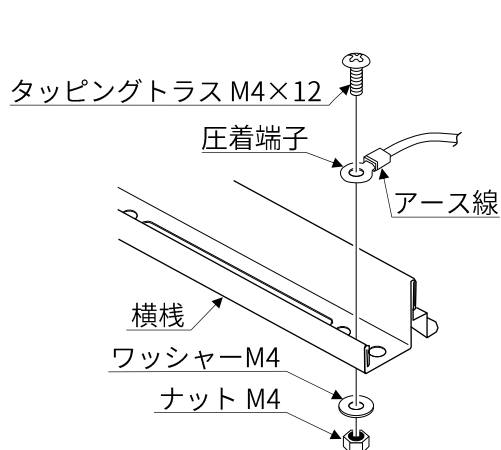
図 4-1. YSⅡでの架台のアース接続
