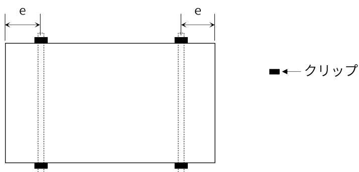
図7. 4箇所以上で固定する場合 (レールと長辺枠が垂直)
