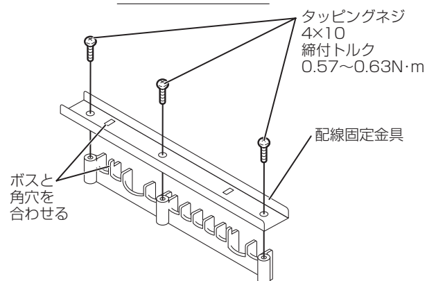
配線固定方法と位置
