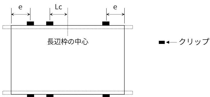
図 10. 6 箇所以上で固定する場合 (レールと長辺枠が平行)
