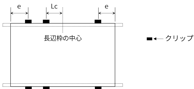
図 10. 6 箇所以上で固定する場合 (レールと長辺枠が平行)
