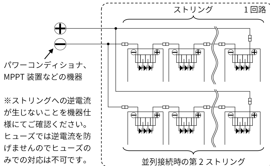
図 12. 2 本のストリングを並列接続する場合
