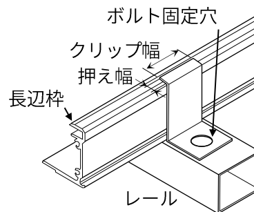
図 6-b. レールと長辺枠が垂直の場合
