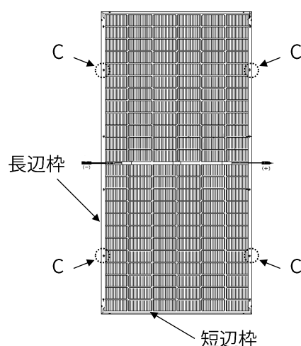
図4. モジュール裏面図
