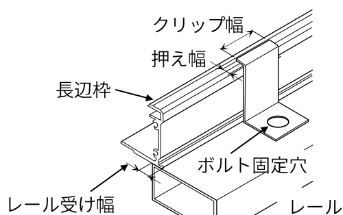
図 6-a. レールと長辺枠が平行の場合
