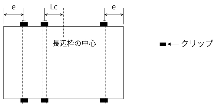
図 9. 6 箇所以上で固定する場合 (レールと長辺枠が垂直)
