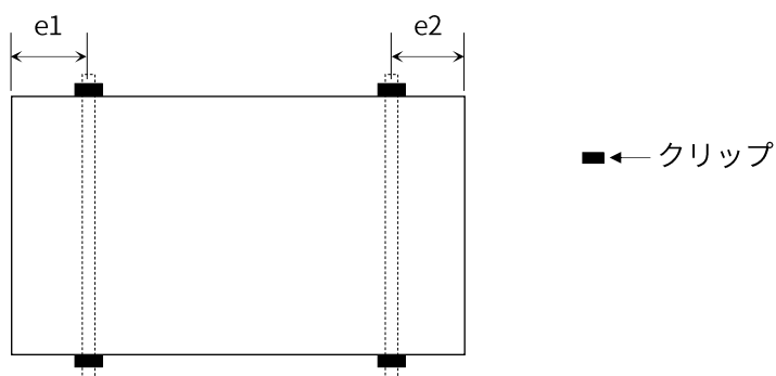
図7. 4箇所以上で固定する場合 (レールと長辺枠が垂直)
