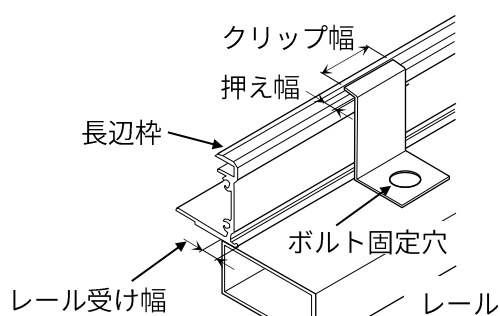
図 6-a. レールと長辺枠が平行の場合
