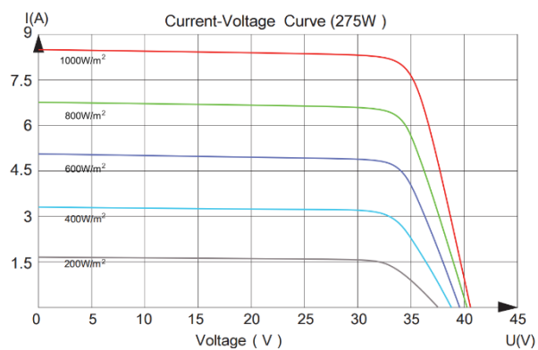
図 12. モジュールの低照度特性(I-V)
