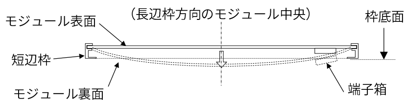
図3. モジュールのたわみ模式図（側面）
