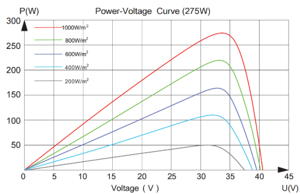
図 13. モジュールの低照度特性(P-V)
