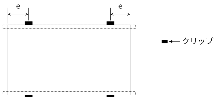
図8. 4箇所以上で固定する場合 (レールと長辺枠が平行)
