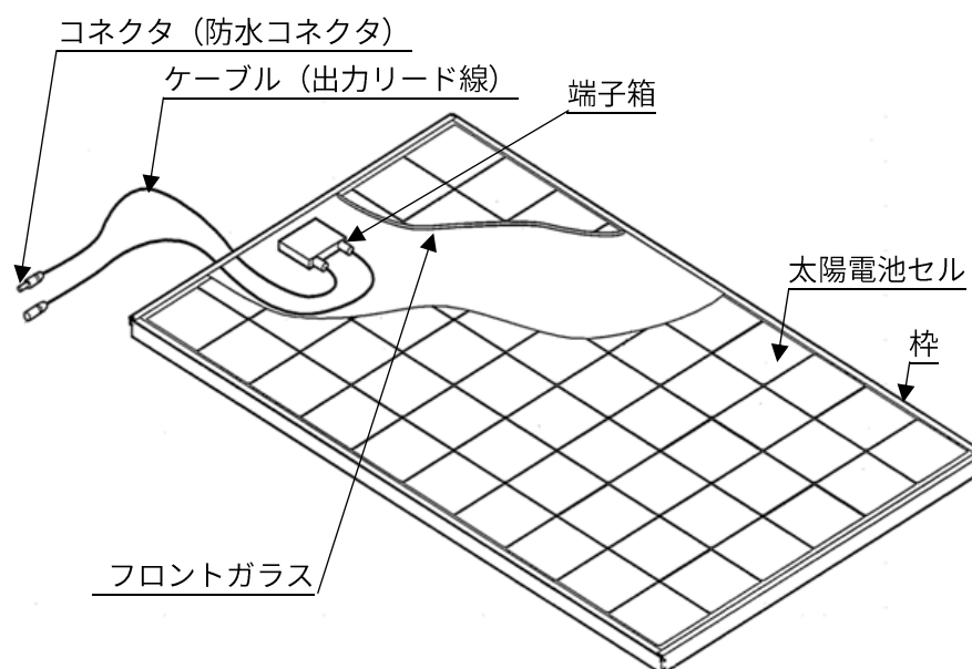
図 1. 太陽電池モジュール構成図
