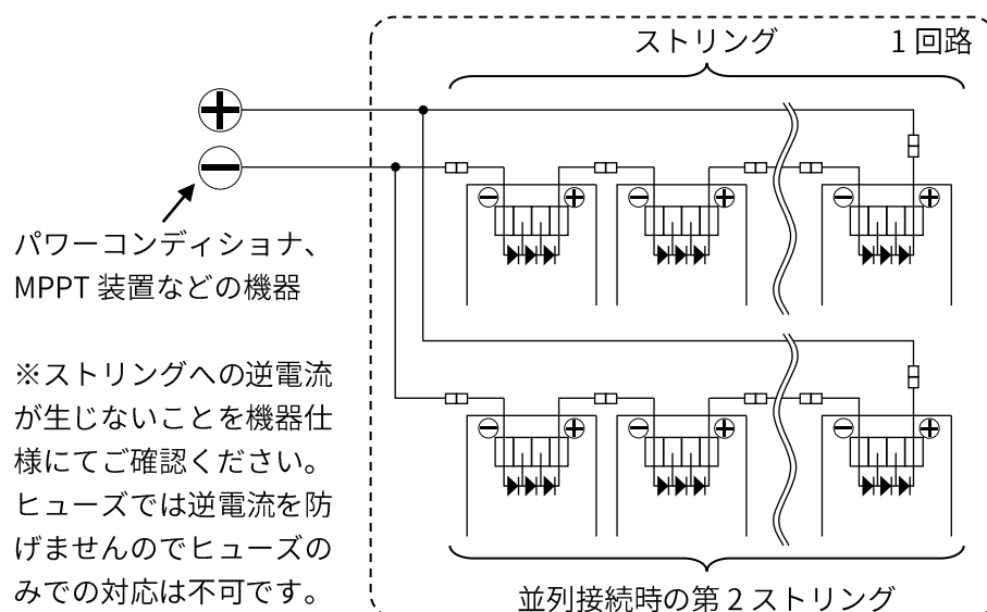
図 6. 2 本のストリングを並列接続する場合
