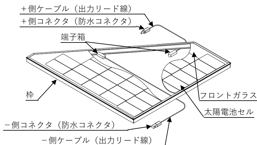
図 1. 太陽電池モジュール構成図
