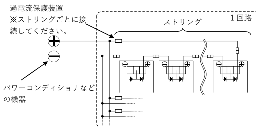
図 6. 3 本以上のstringを並列接続する場合
