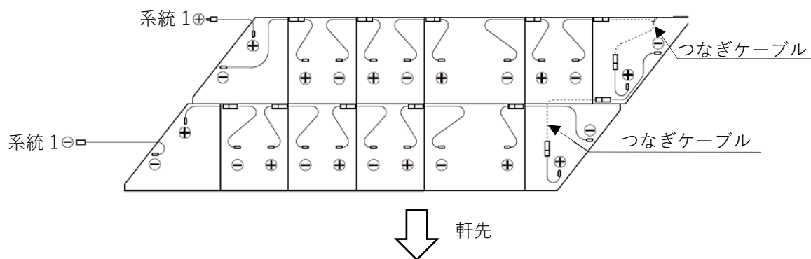
図 3-12. つなぎケーブルの接続例
