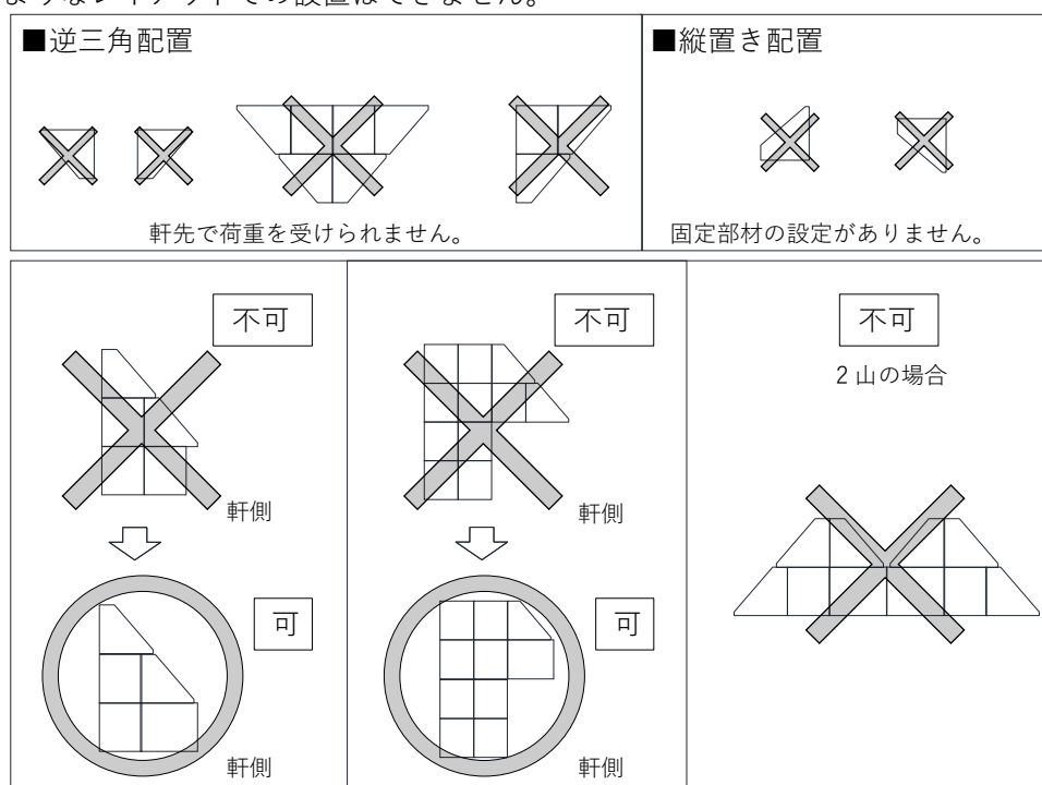
図 3-13. 禁止レイアウト
