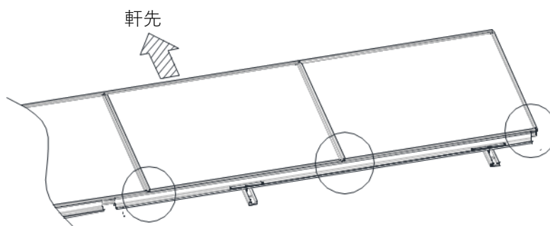
図 3-8. YSⅢ工法 モジュール固定手順
