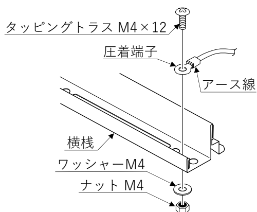
図 4-2. YS II での架台のアース接続
