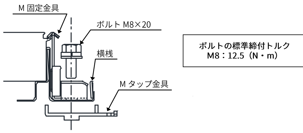
図 3-3. YS II 工法 金具の固定図
