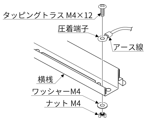
図 4-1. YSⅡでの架台のアース接続
