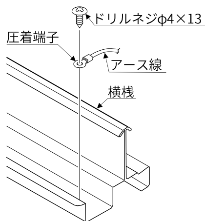
図 4-2. YSⅢでの架台のアース接続
