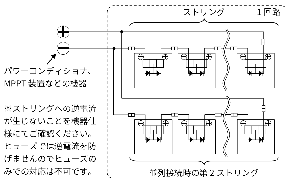
図 6. 2 本のストリングを並列接続する場合
