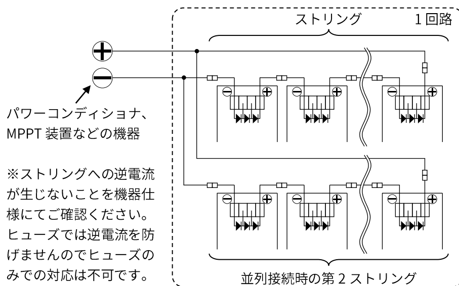
図 12. 2 本のstring を並列接続する場合
