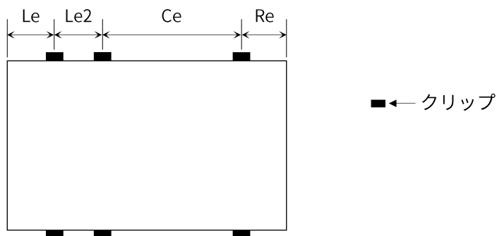
図 8. 6 カ所で固定する場合
