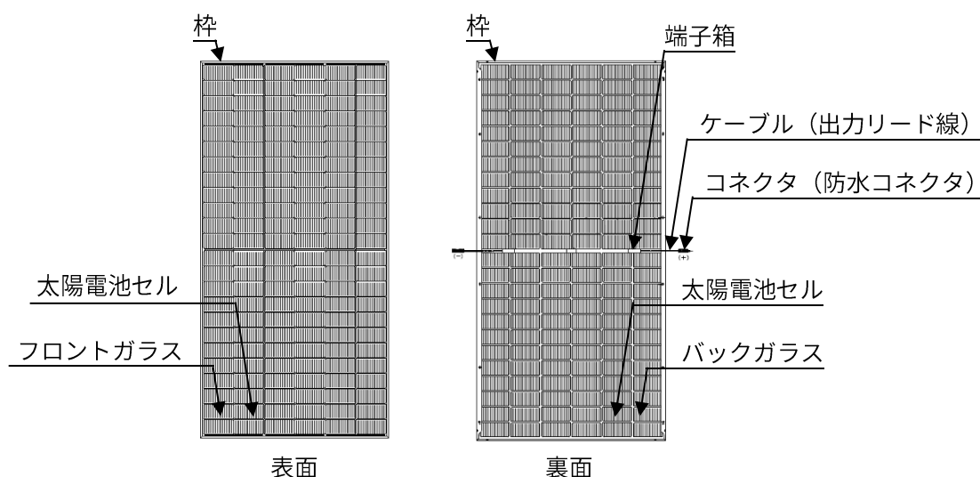
図 1. 太陽電池モジュール構成図
