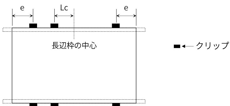
図 10. 6 カ所で固定する場合 (レールと長辺枠が平行)
