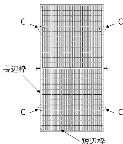
図4. モジュール裏面図
