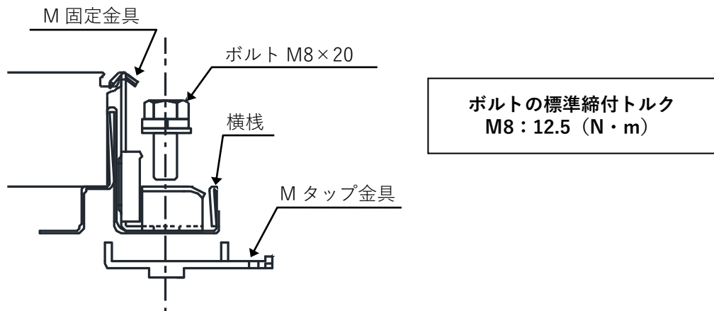
図 3-5. YS II 工法 金具の固定図
