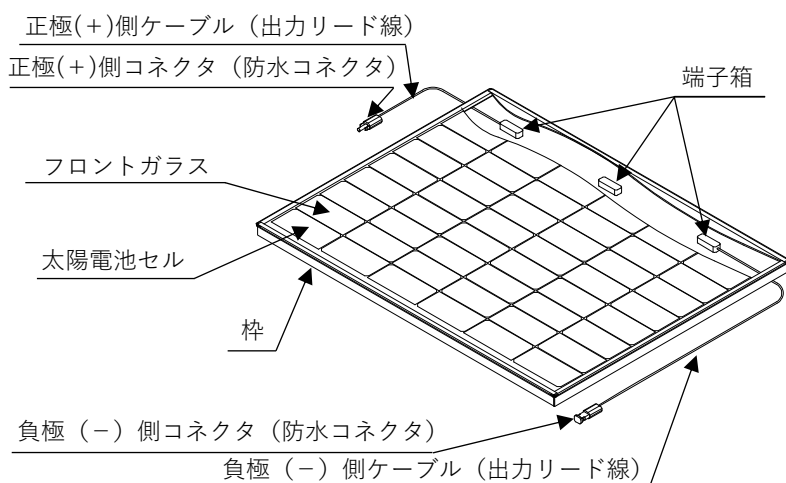
図 1. 太陽電池モジュール構成図
