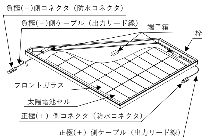
図 1. 太陽電池モジュール構成図
