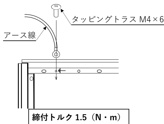
図 4-1. モジュール枠での架台のアース接続
