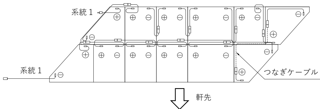
図 3-12. つなぎケーブルの接続例
