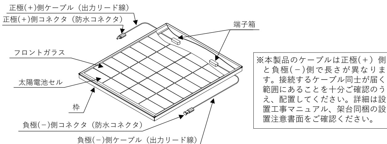
図 1. 太陽電池モジュール構成図
