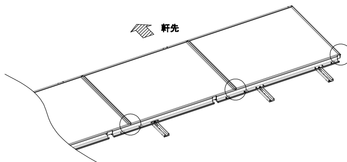
図 3-8. YSⅢ工法 モジュール固定手順
