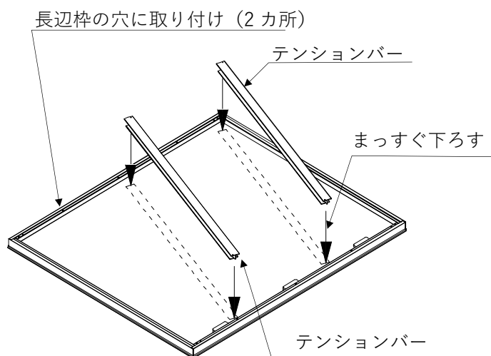
図 3-18. テンションバーの取り付け
