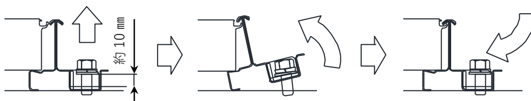
図 3-7. YSⅢ工法 モジュール固定手順
