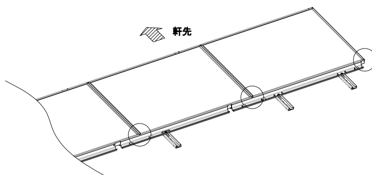
図 3-8. YSⅢ工法 モジュール固定手順
