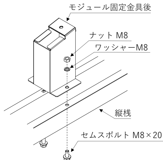
図 3-13. 折板屋根工法 金具後の固定図
