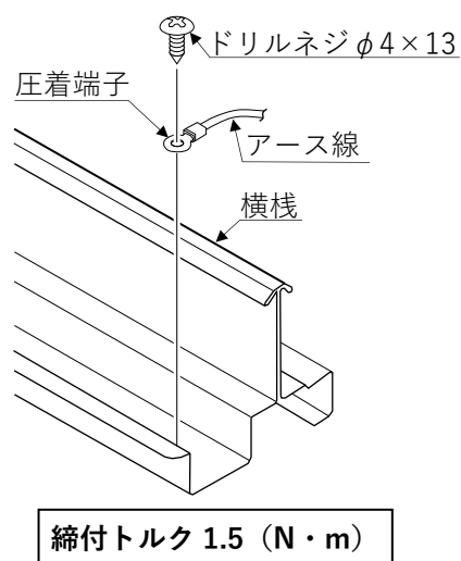
図 4-3. YS III での架台のアース接続
