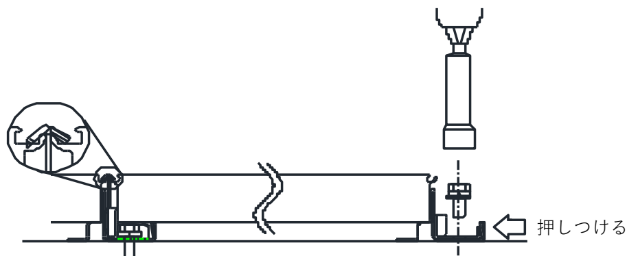
図 3-4. YS II 工法 モジュール固定図
