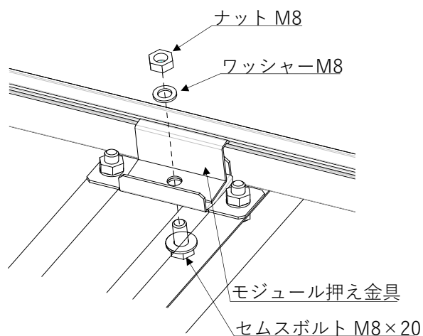
図 3-16. 折板屋根工法 軒先側
