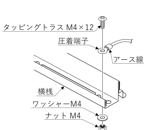
図 4-2. YS II での架台のアース接続
