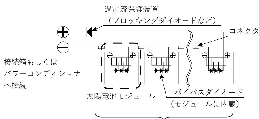
図2. 太陽電池モジュールの配線構成例
