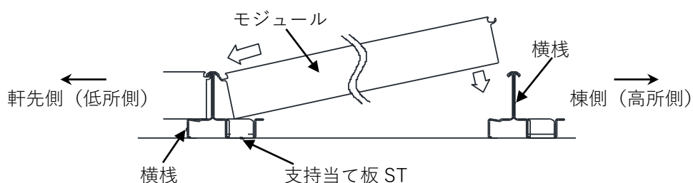
図 3-6. YSⅢ工法 モジュール固定図
