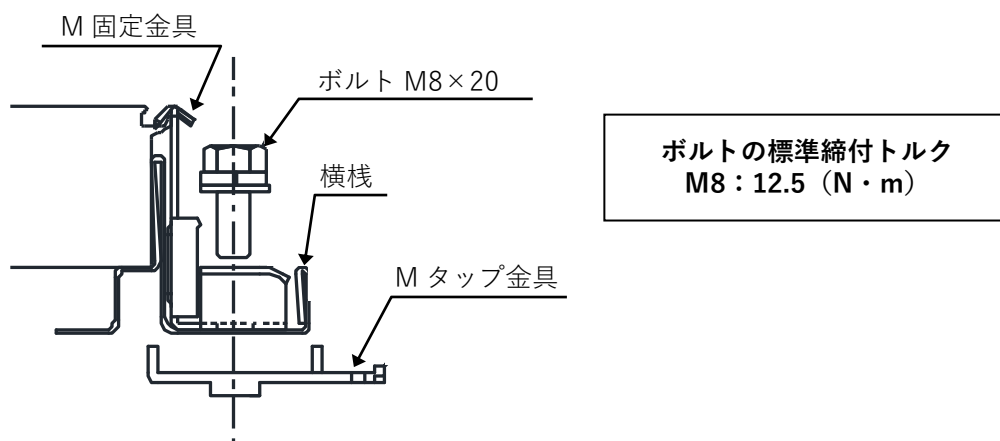
図 3-5. YS II 工法 金具の固定図
