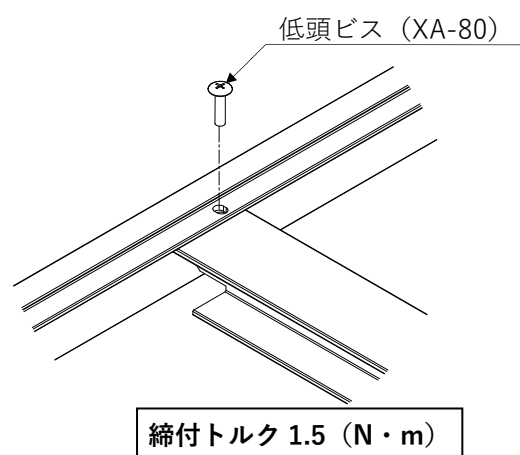
図 3-19. テンションバーの取り付け部拡大図
