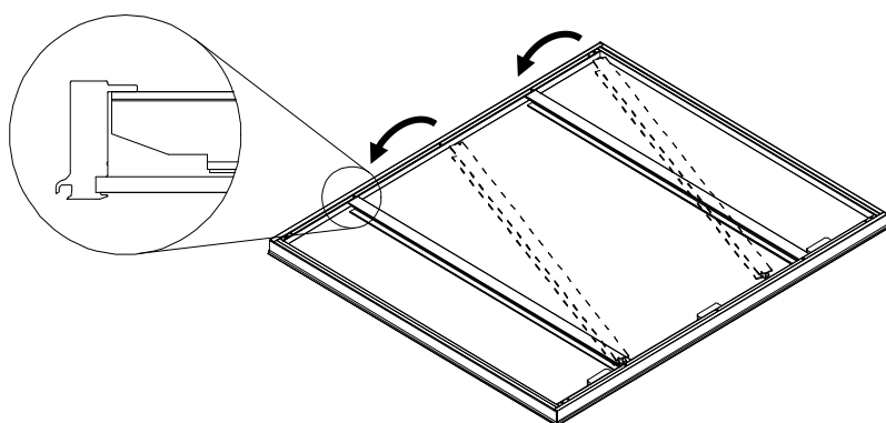
図 3-20. テンションバー取り付け完成図
