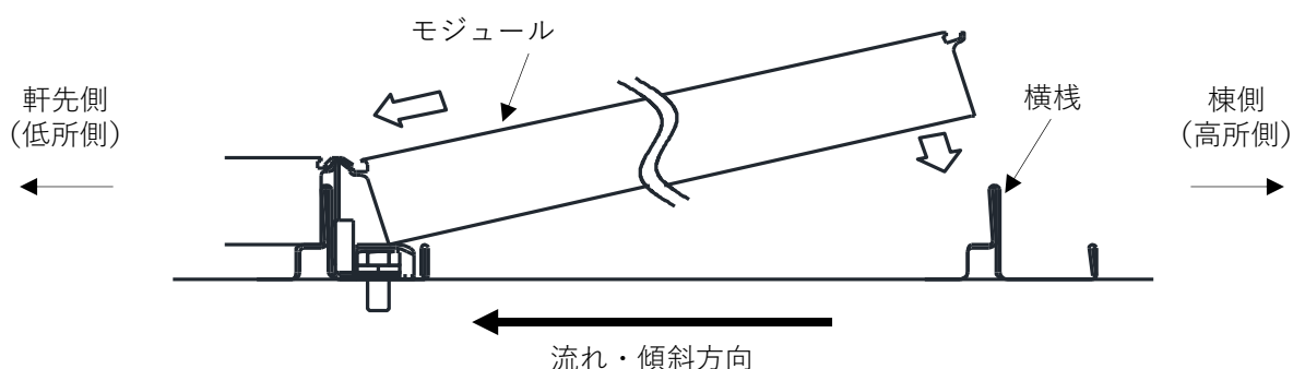
図 3-3. YS II 工法 モジュール固定図
