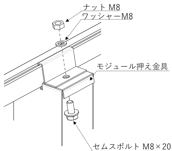
図 3-17. 折板屋根工法 棟側
